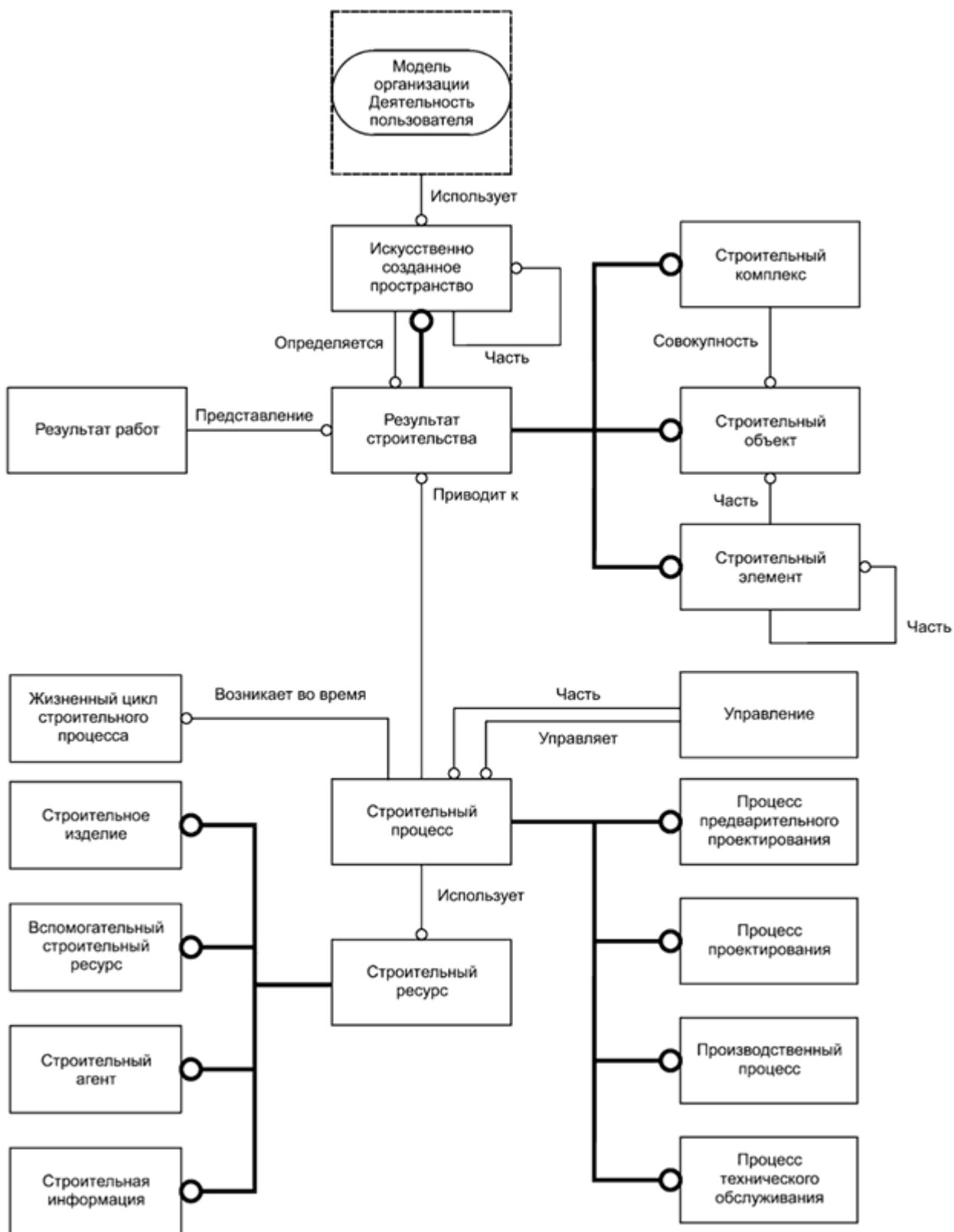
Рисунок 1 - Классы и их основные взаимосвязи На схеме используются обозначения в упрощенном формате EXPRESS-G.
