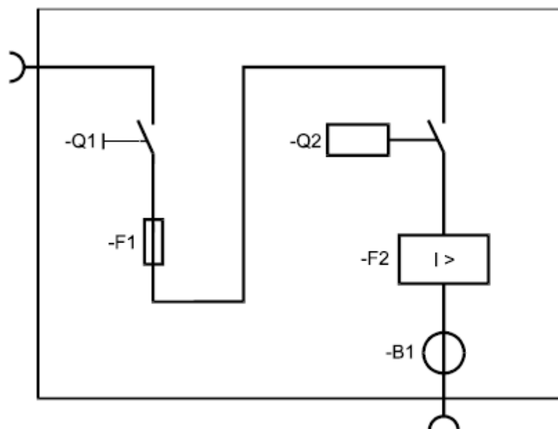
а) Принципиальная схема
