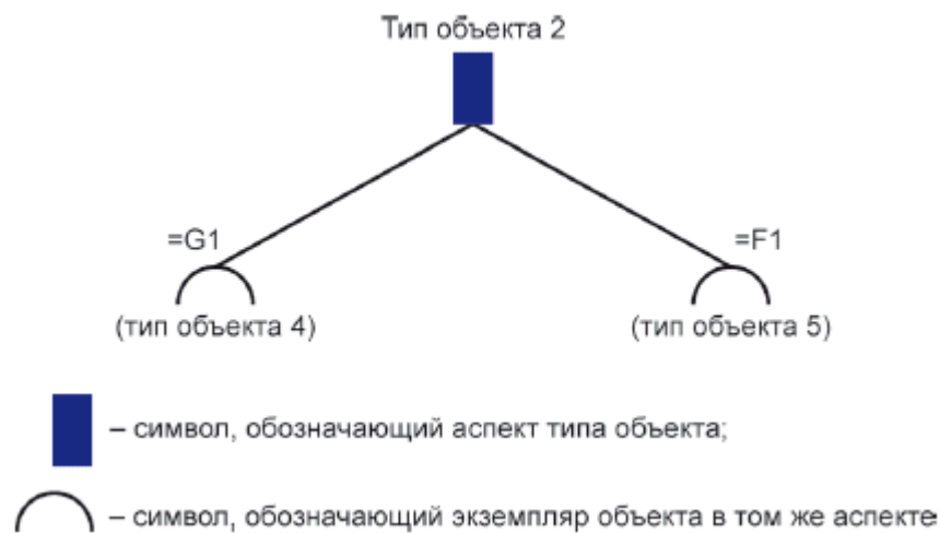
Рисунок G.2 - Функционально-ориентированная структура типа объекта 2
