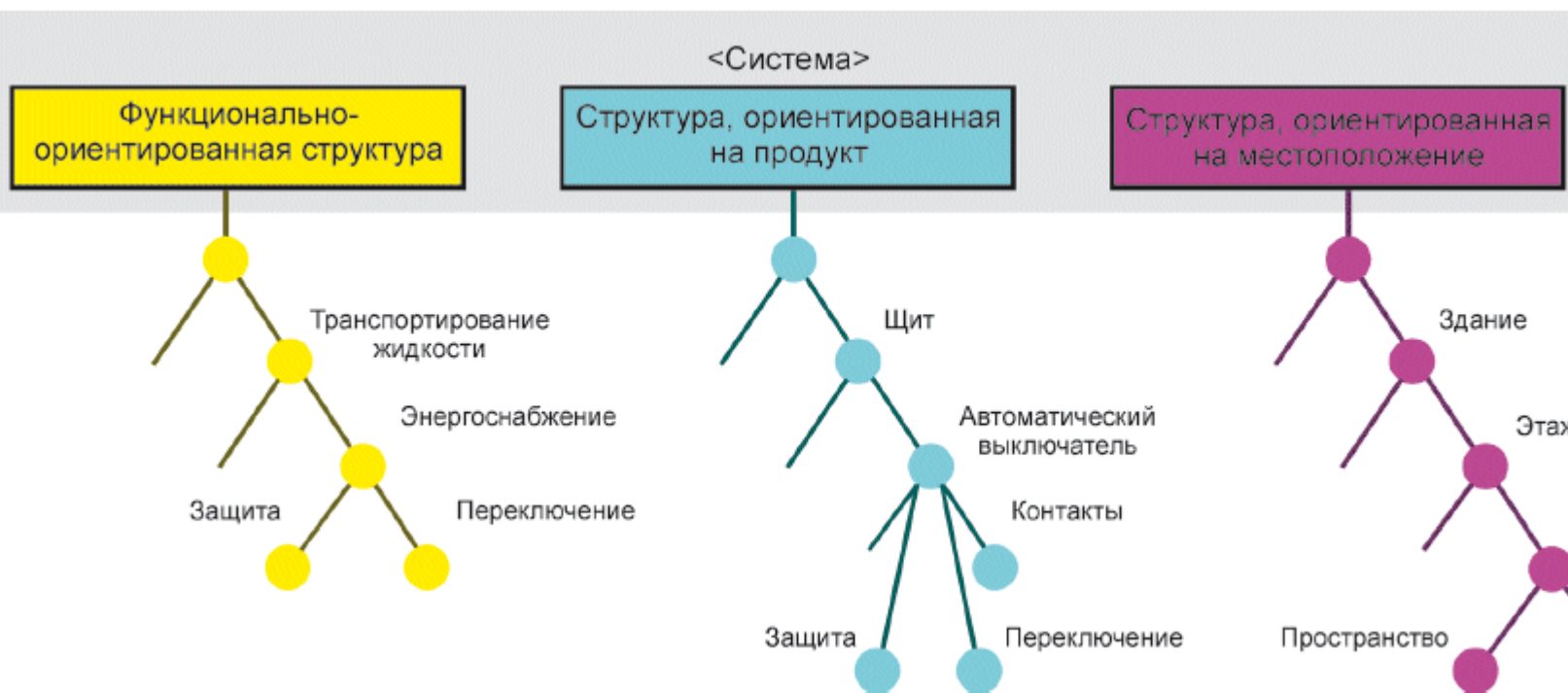
Рисунок С.8 - Завершенные структуры технической системы
