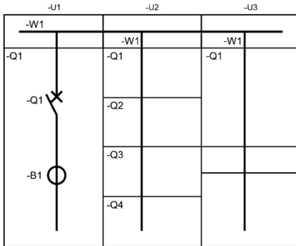
Рисунок Н.4 - Компоновочный чертеж компонентов ЩСУ =G1=W1
