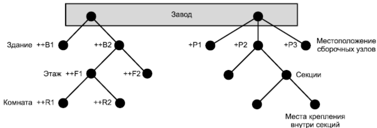
Рисунок F.4 - Структуры завода, ориентированные на местоположение Системы кодовых обозначений для трех сборочных узлов могут быть следующими:
