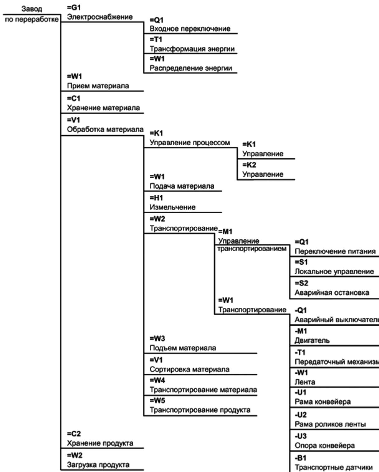
Рисунок Н.3 - Древоподобная структура для частей установки по обработке материалов
