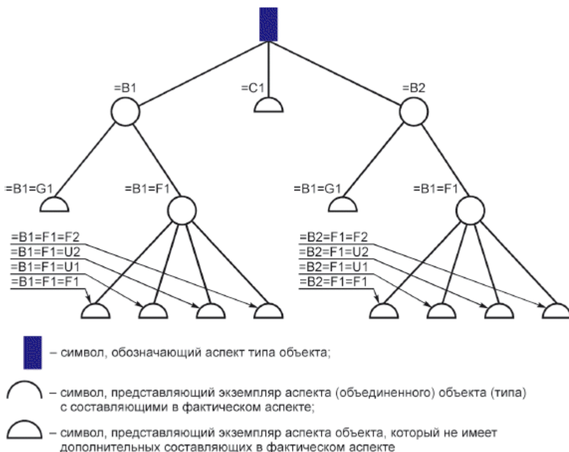
Рисунок G.4 - Объединенная функционально-ориентированная структура типа объекта 1 Приложение Н (справочное)
