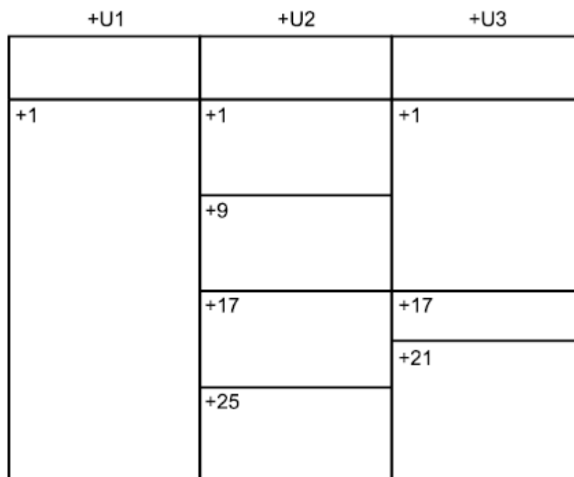
Рисунок Н.5 - Компоновочный чертеж местоположений ЩСУ =G1=W1
