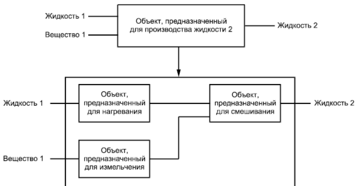
Рисунок 4 - Функция и ее подфункции
