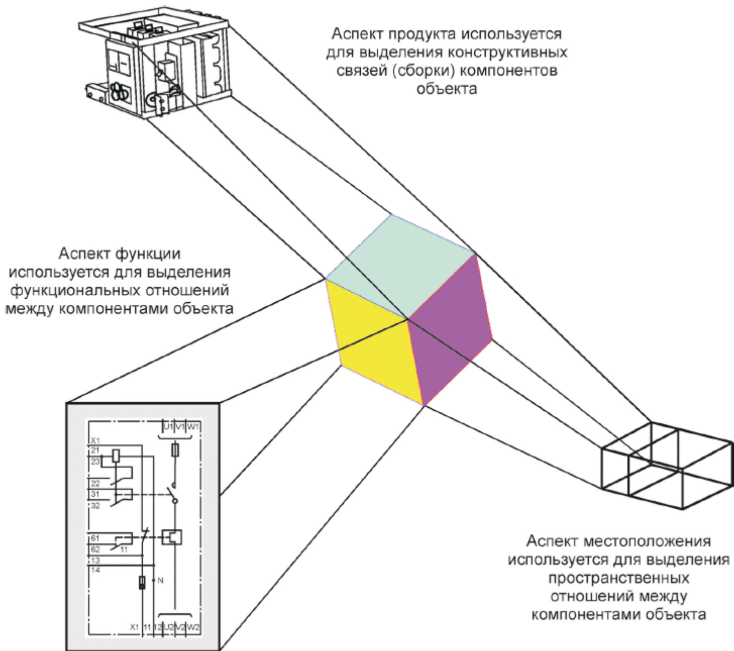
Рисунок 3 - Аспекты объекта
