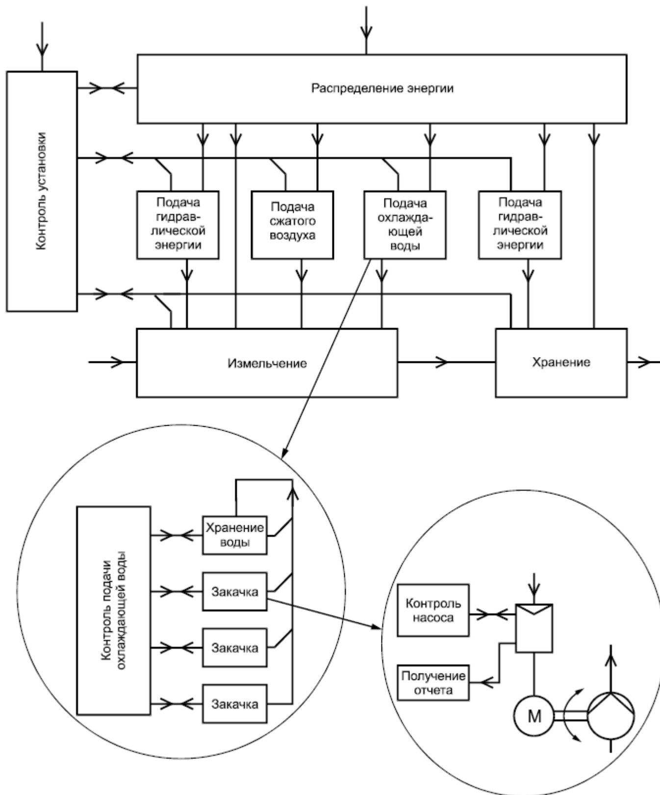
Рисунок 14 - Функционально-ориентированная структура
