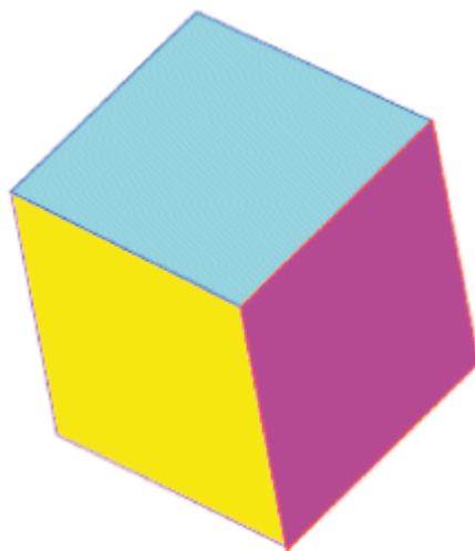
Рисунок 2 - Объект
