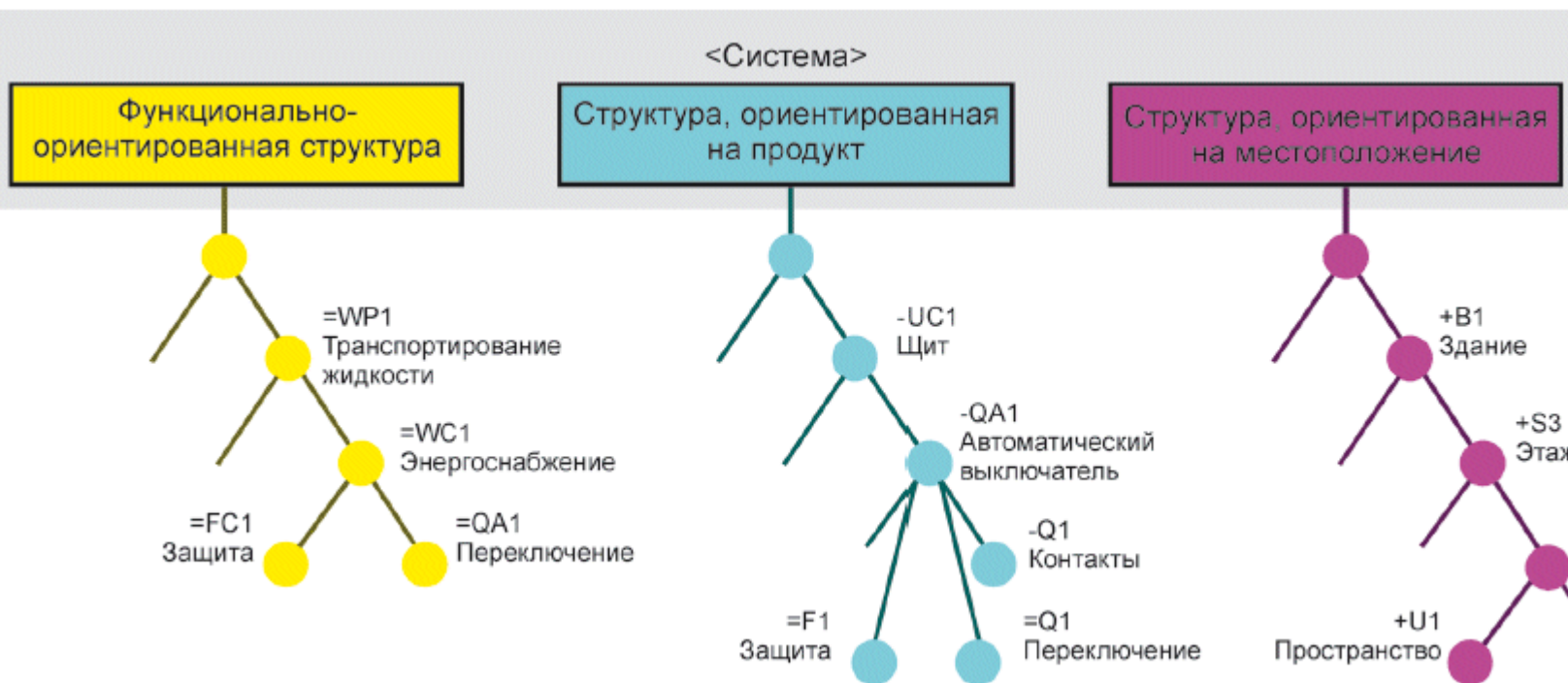
Рисунок С.9 - Структуры с обозначенными подобъектами
