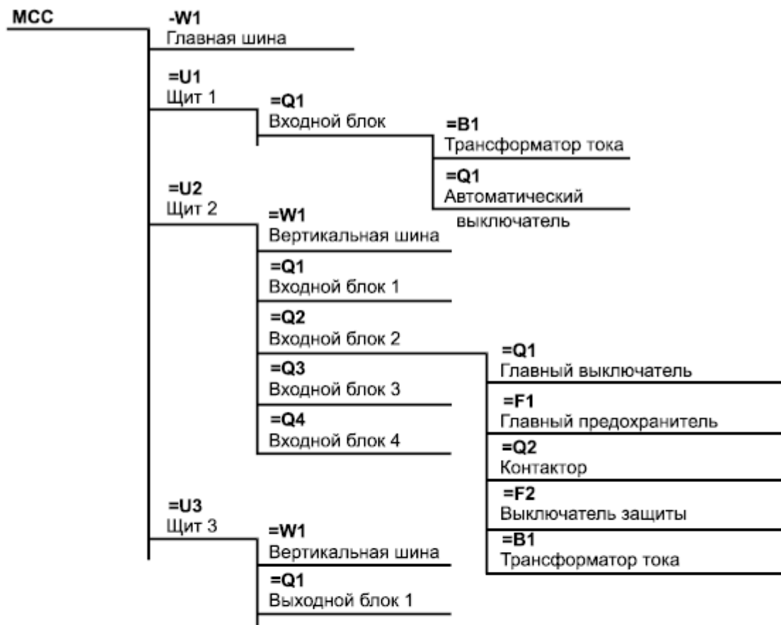
а) Древоподобная структура, ориентированная на продукт
