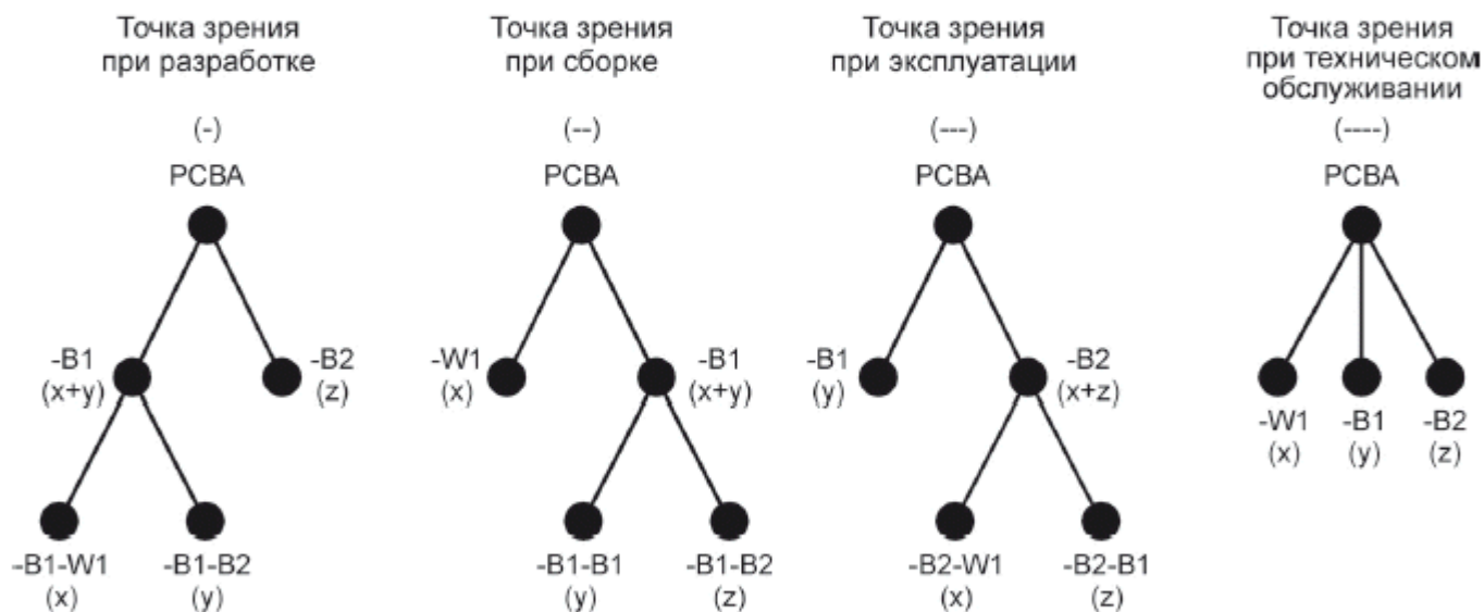
б) Четыре возможных структуры, ориентированные на продукт
