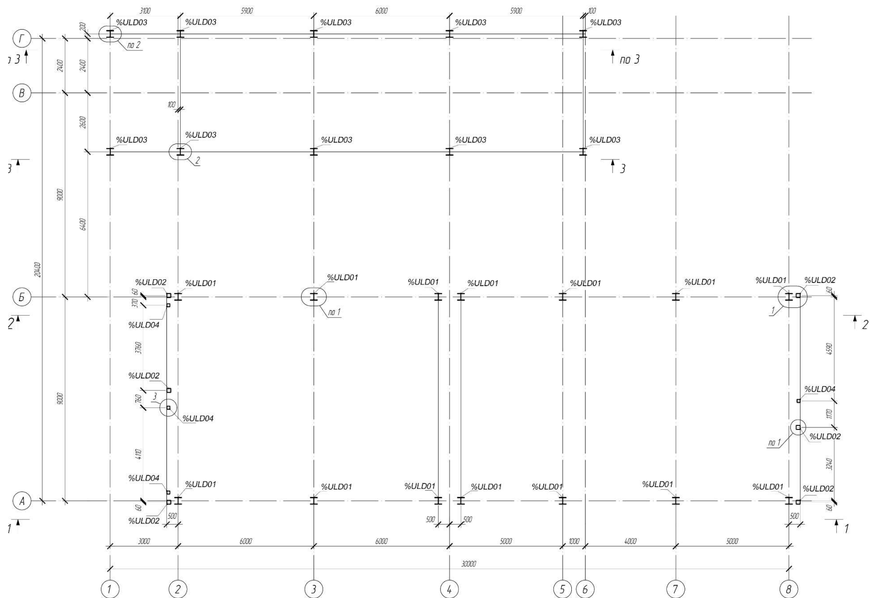
Рисунок Б.5.2 – Обозначение элементов несущего каркаса ЛОС на разрезе
