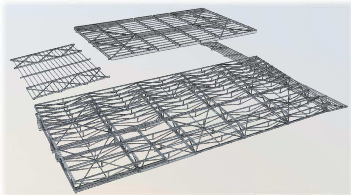
Рисунок А.11 – Подсистема «Балочные конструкции крыши» системы «Конструкции плоской крыши»
