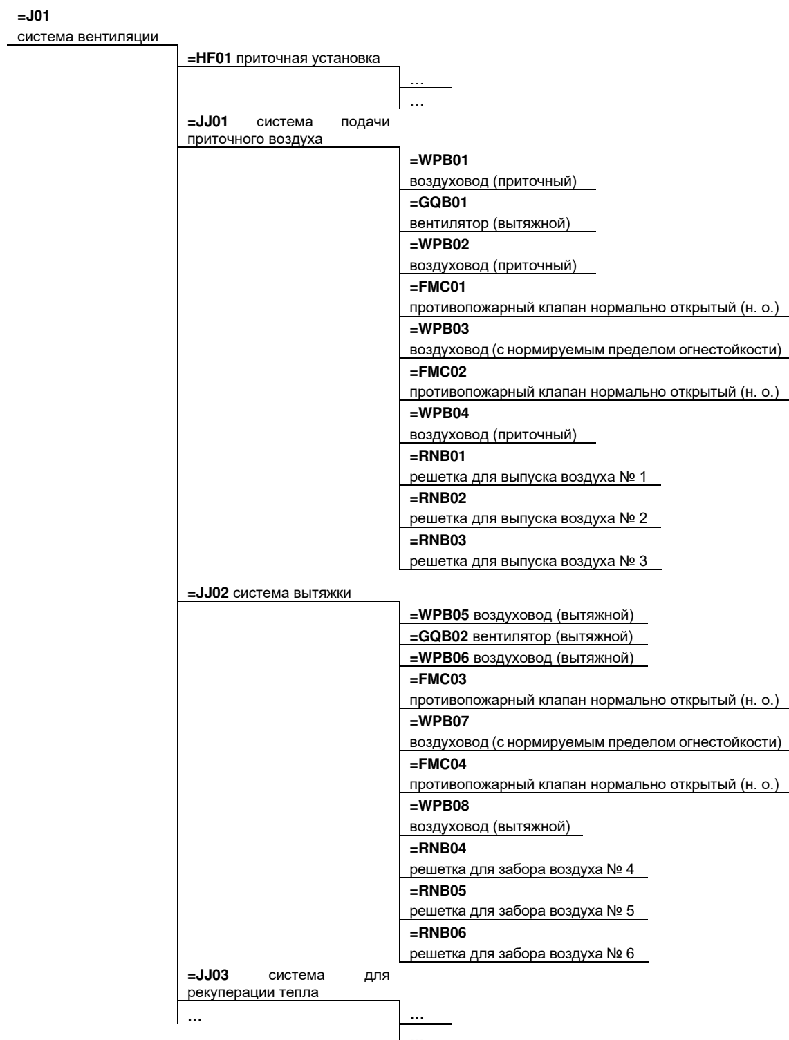
Рисунок Б.2.2 – Фрагмент схемы иерархической структуры представления системы вентиляции машинного цеха
