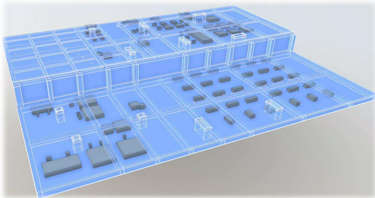
Рисунок А.5 – Подсистема «Конструкции комбинированных фундаментов» системы «Фундамент» <TeS>-A01.AB01/%%A20.AB50
