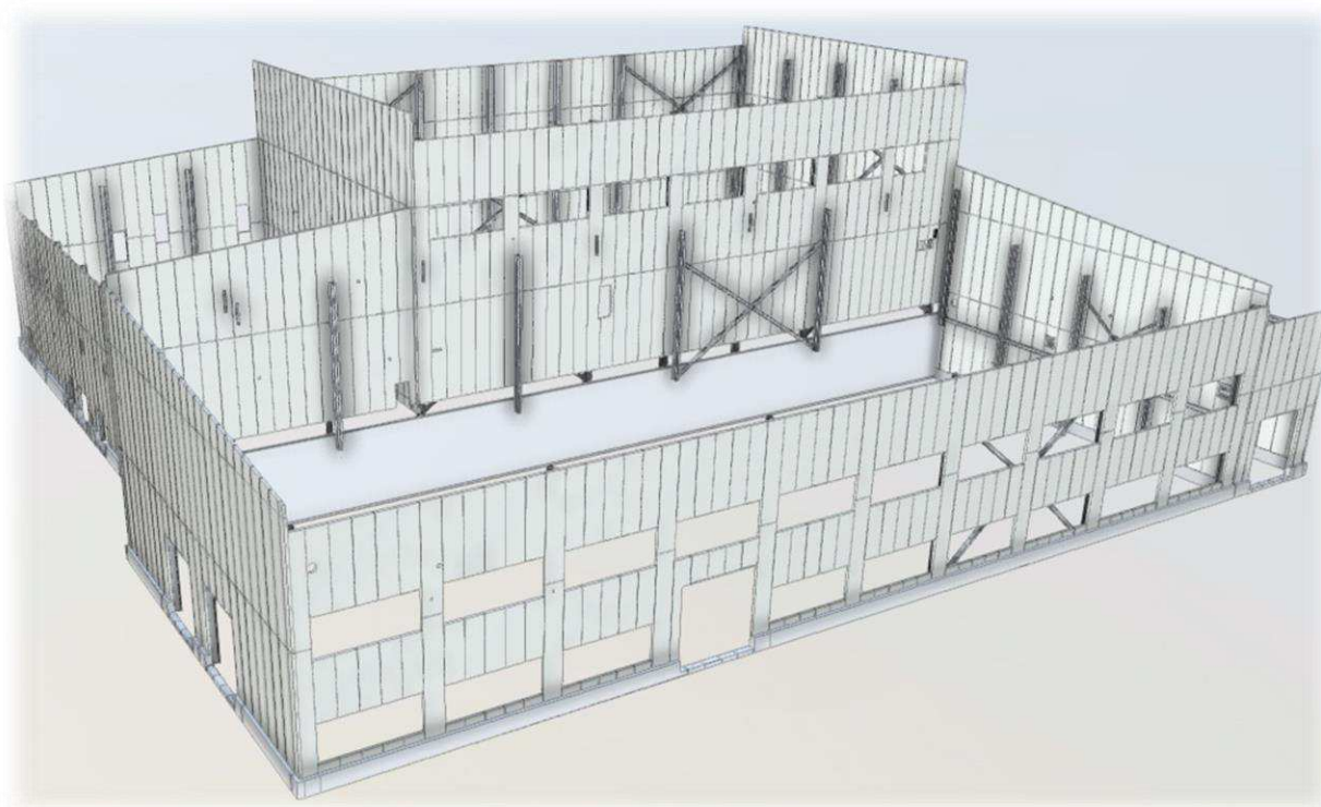
Рисунок А.7 – Подсистема «Конструкции стен со стойками» системы «Система наружных стен»
