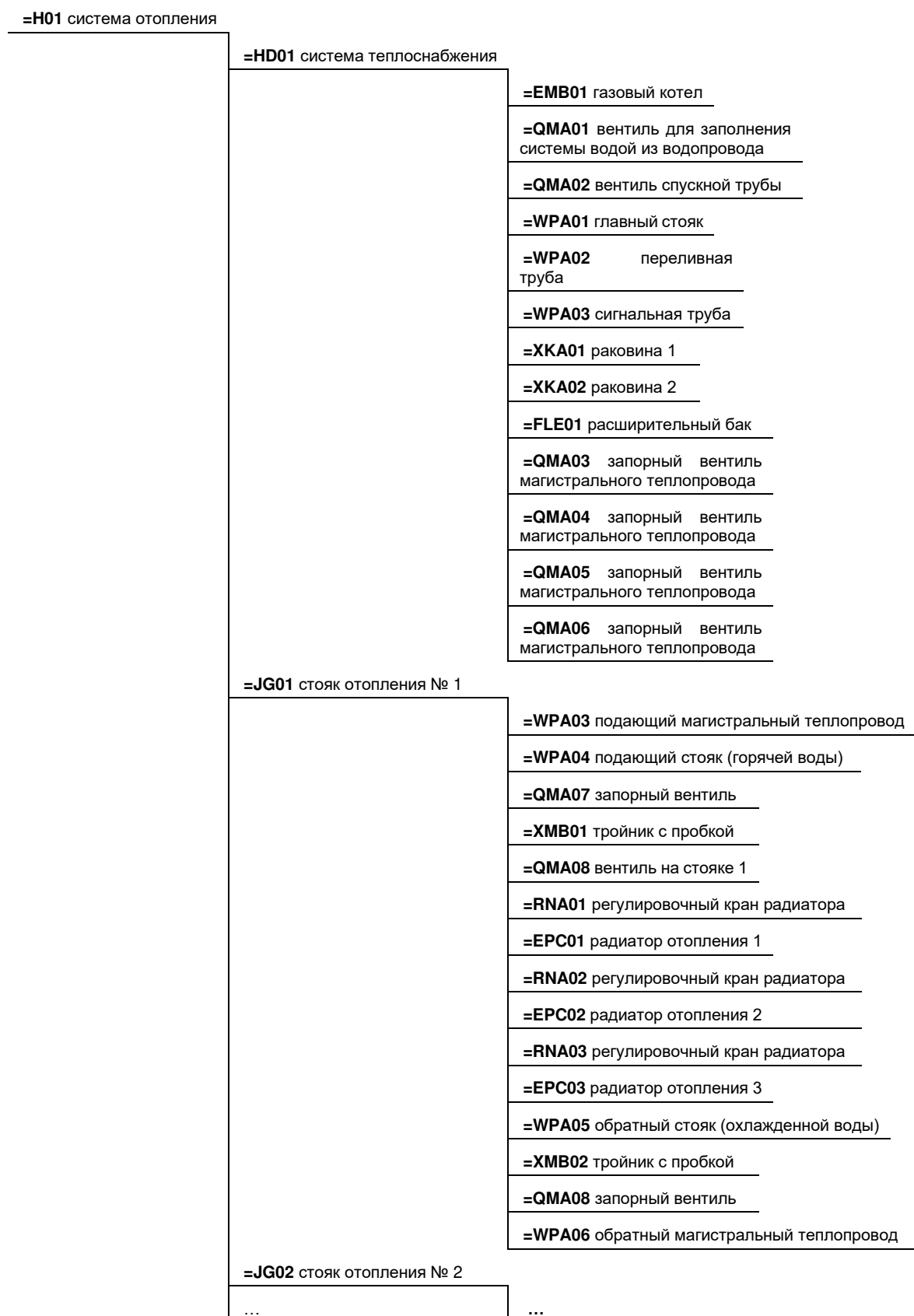
Рисунок Б.1.2 – Схема иерархической структуры представления системы отопления административного здания
